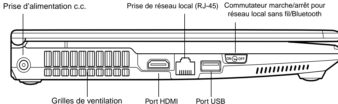
Figure 3. Côté gauche de l'ordinateur LifeBook
