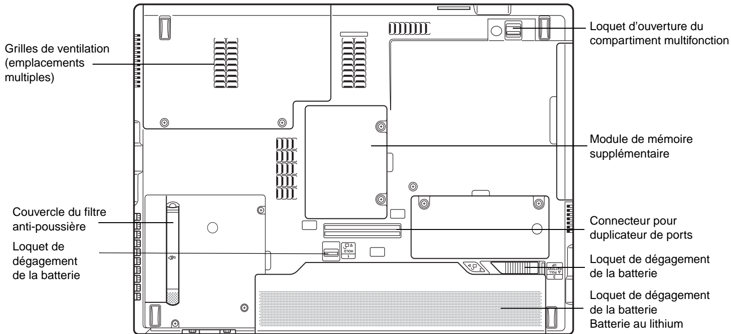
Figure 6. Dessous de l'ordinateur portable LifeBook
