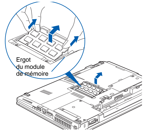
Figure 34. Retrait d'un module de mémoire
