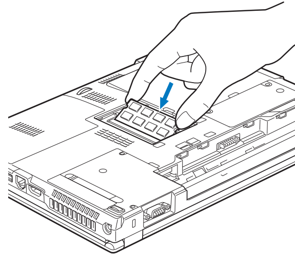
Figure 33. Installation d'un module de mémoire
