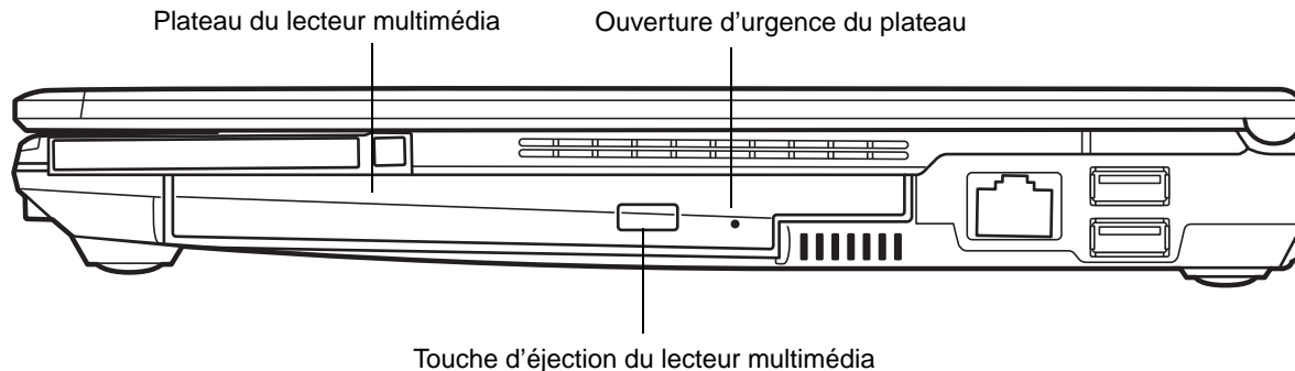
Figure 27. Lecteur optique
