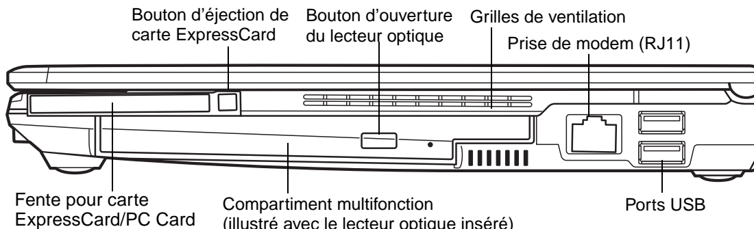
Figure 4. Côté droit de l'ordinateur LifeBook
